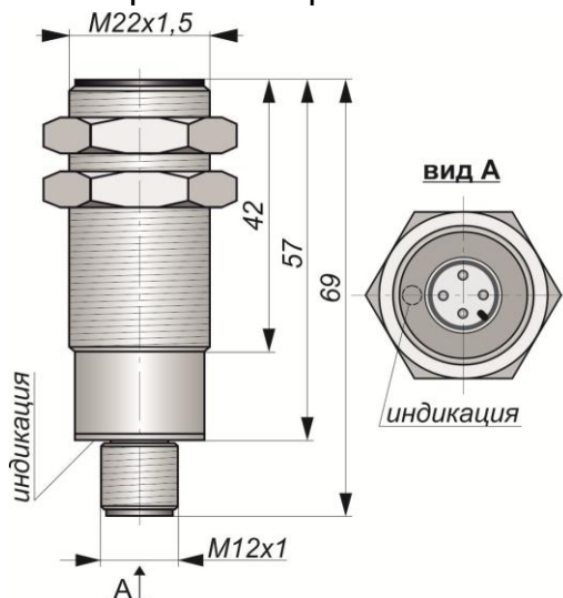
Габаритный чертеж
